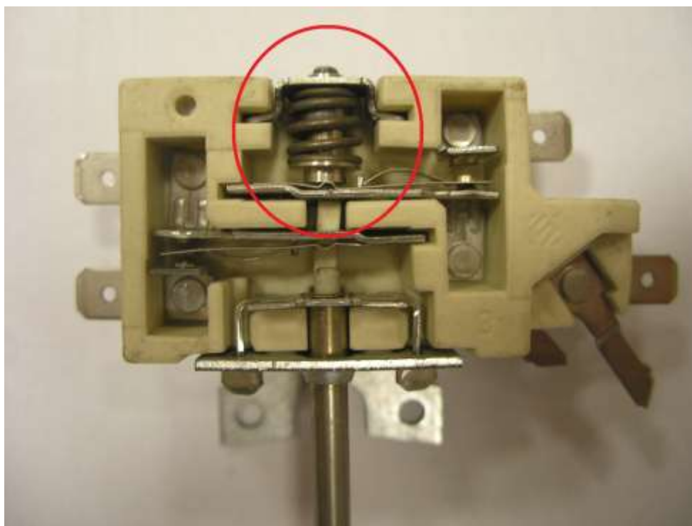
Slika 6. Pozicija i primjena čahure, opruge i ležaja u štapnom limiteru
