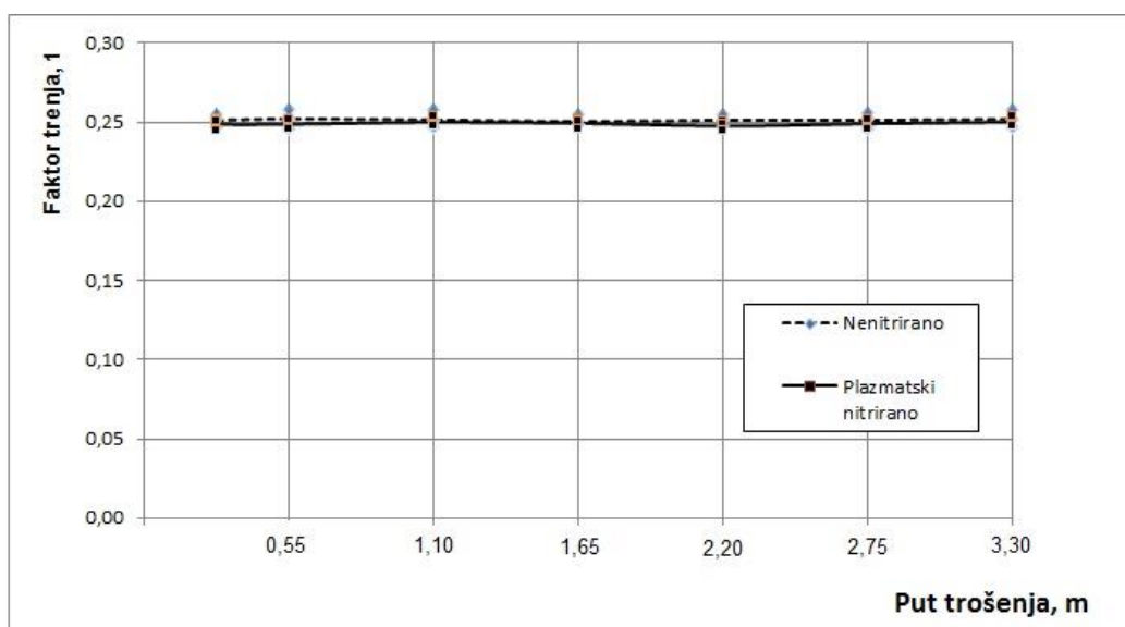
Slika 41 Promjena faktora trenja nitrirane i nemitrirane legure Ti6Al4V ovisno o putu trošenja na uređaju s kliznim prstenom
