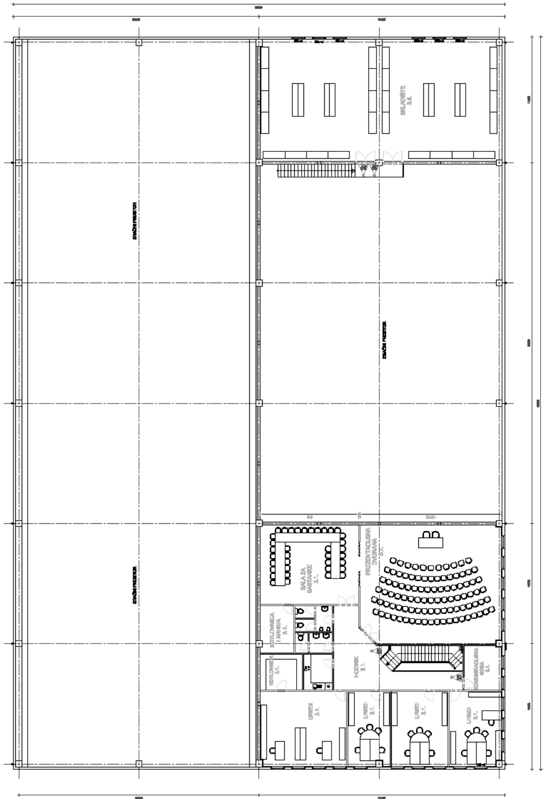
Slika 2.6. Tlocrt kata hale III [3]
