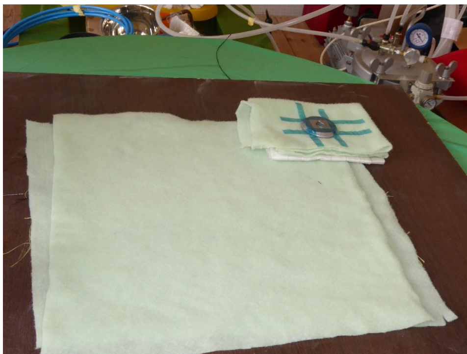
Slika 7.9. Postavljanje tkanine za upijanje viška smole i ventila
