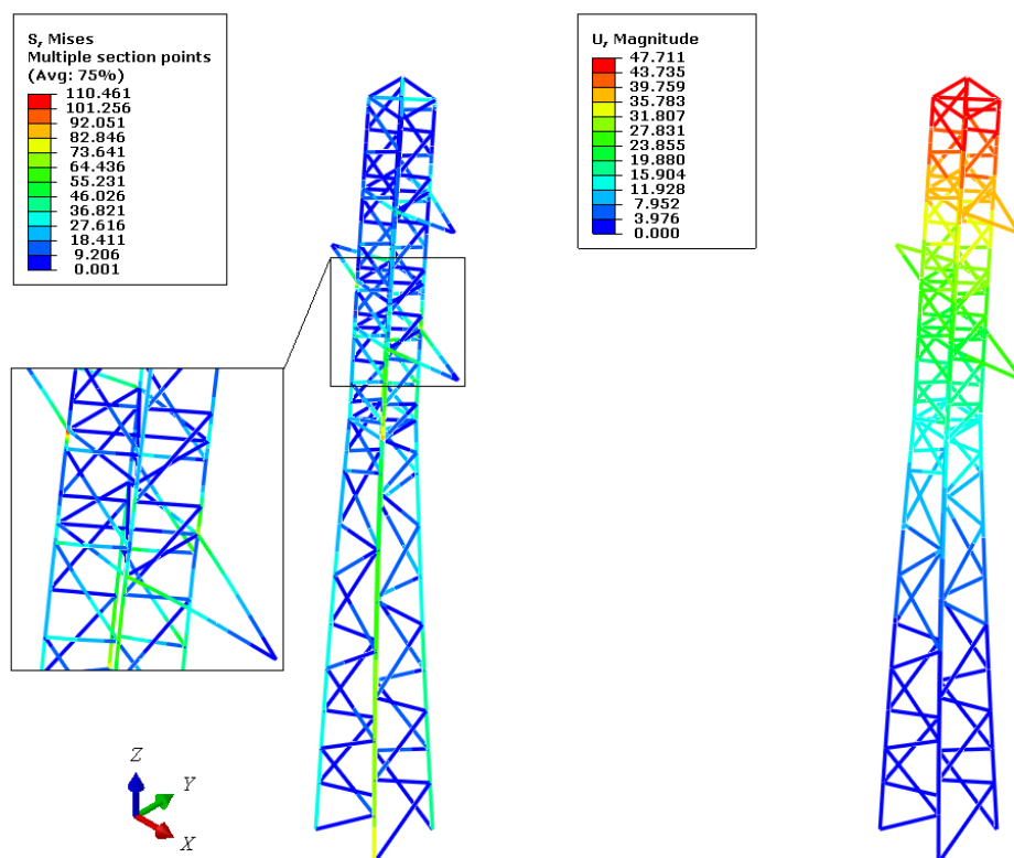
Slika 5.7. Raspodjela napreznja (MPa) i pomaka (mm) za slučaj 68.I.c
