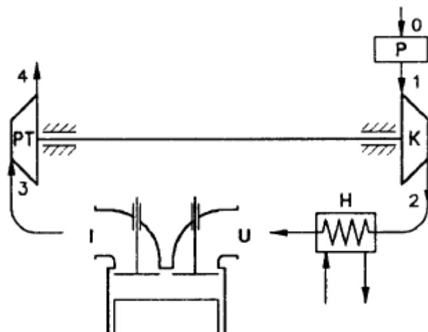
Slika 5. Shema turbonabijanja [2]
