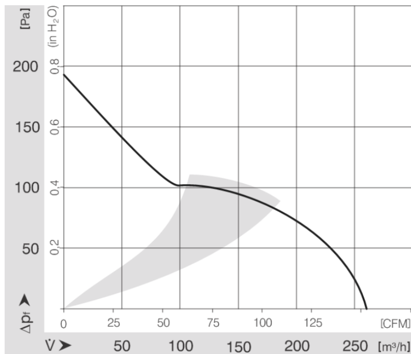
Slika 70. Krivulja 4112 NHH ventilatora
