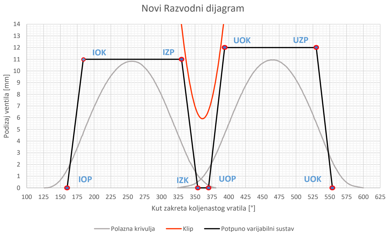
Slika 19. Novi razvodni dijagram
