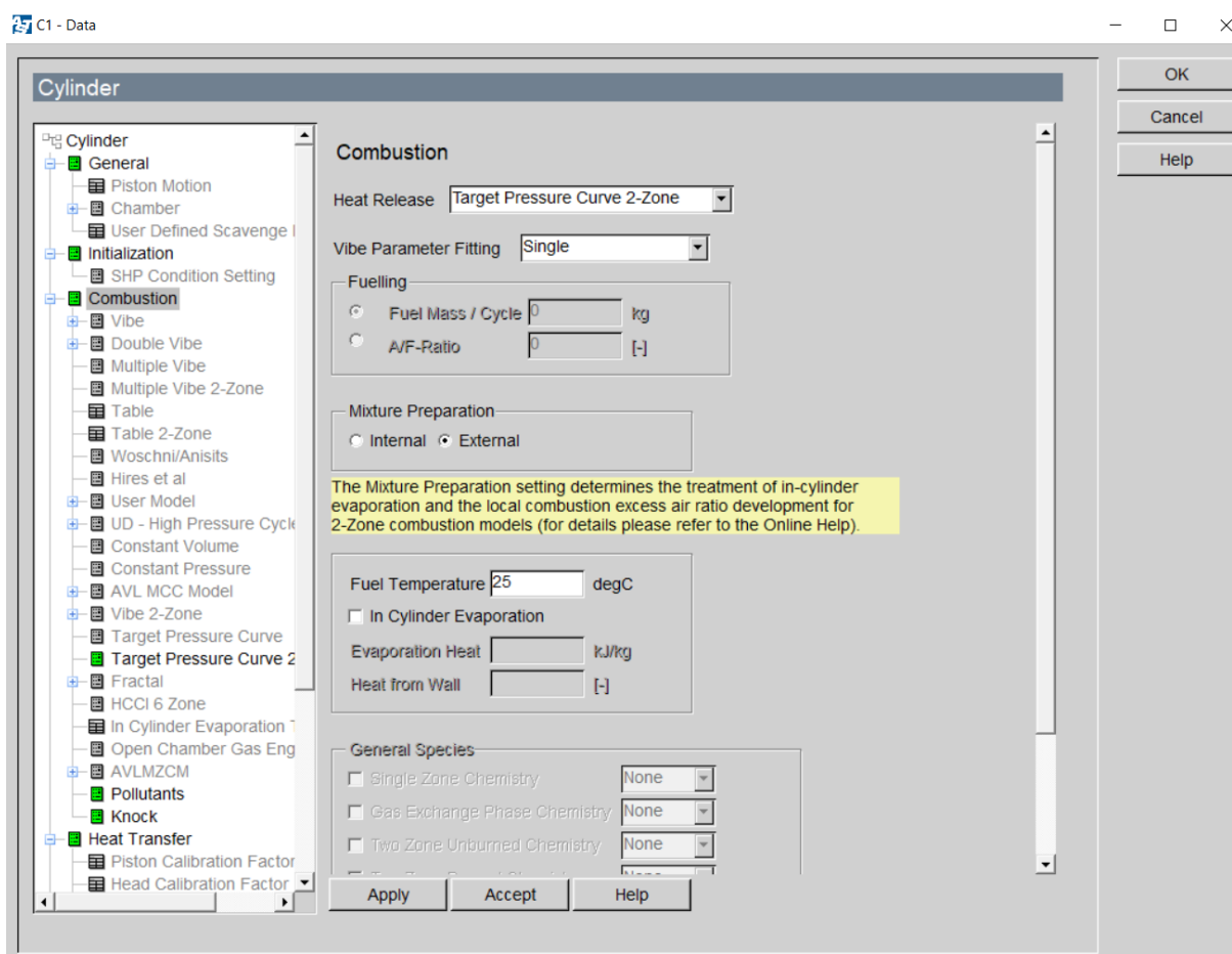
Slika 11. Sučelje "Combustion"
