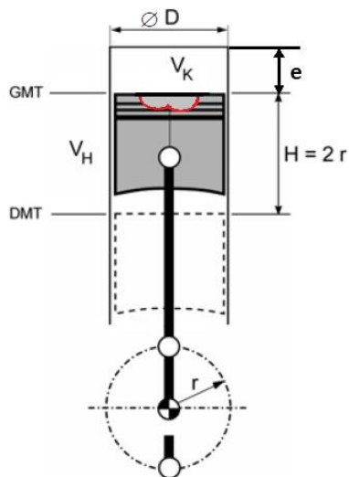
Slika 18. Skica klipa
