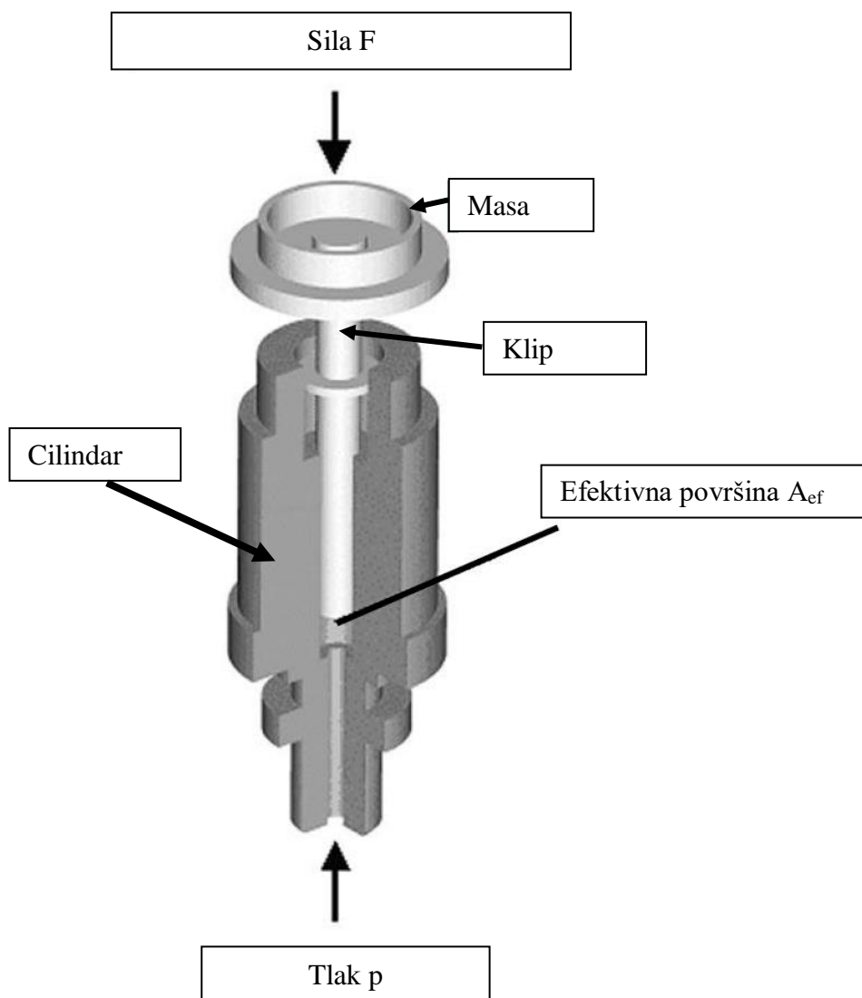
Slika 5. Sklop klip-cilindar [8]
