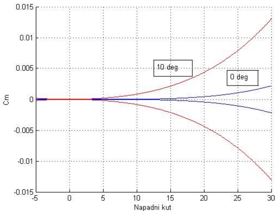
Slika 12. Standardna devijacija koeficijenata momenta propinjanja za različite \delta_e , F-16C
