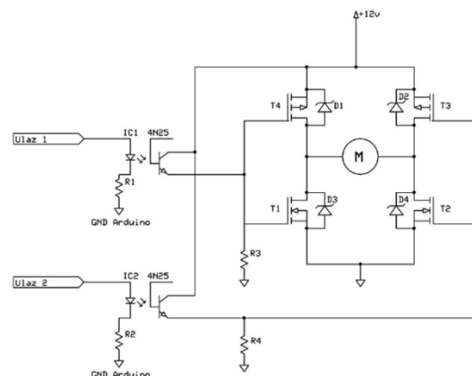
Slika 2.27. Elektronički sklop zaklopke snage Ottovog motora (lijevo), shema elektroničkog sklopa (desno)
