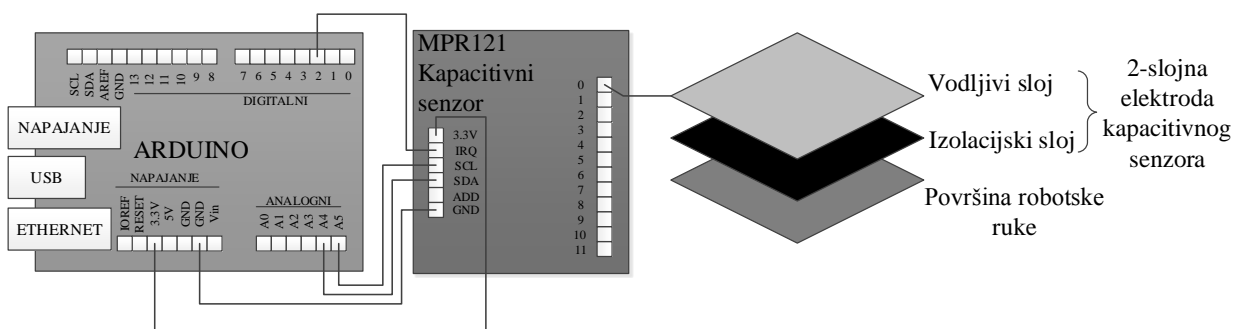
Slika 3.2. Kapacitivni senzor.
