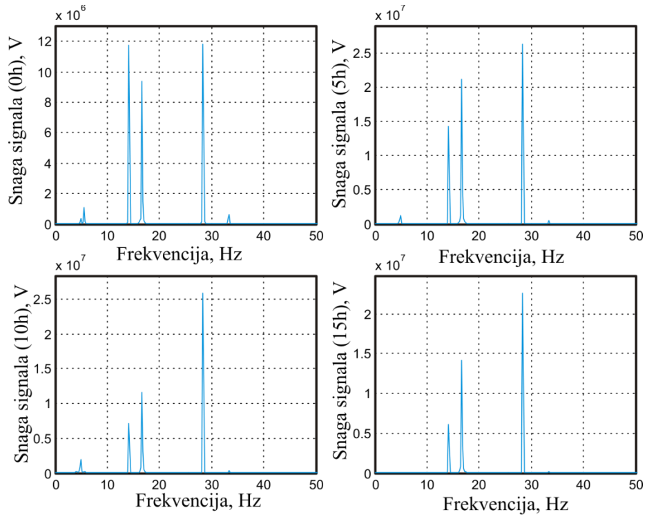
Slika 5.51 FFT analiza filtriranog signala
