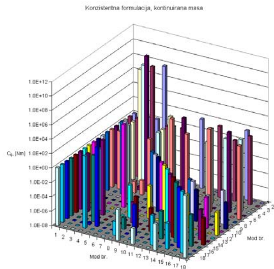
Slika 7-12 Matrica povratne krutosti barže, konzistentna formulacija, (4.3)
