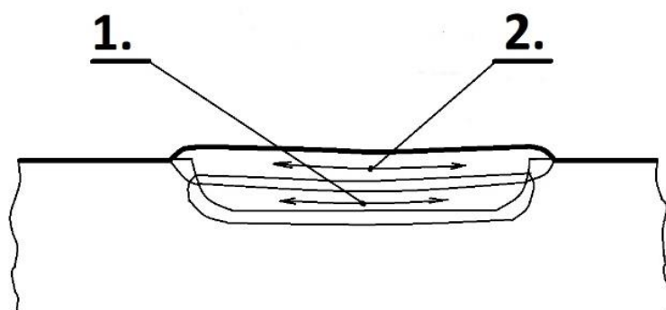
Slika 16 Redoslijed zavarivanja
