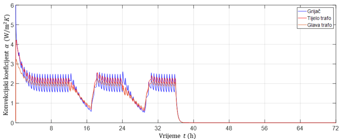
Slika 5.15. Koeficijent prijelaza toplote slobodne konvekcije s zraka na transformatore – slučaj 2
