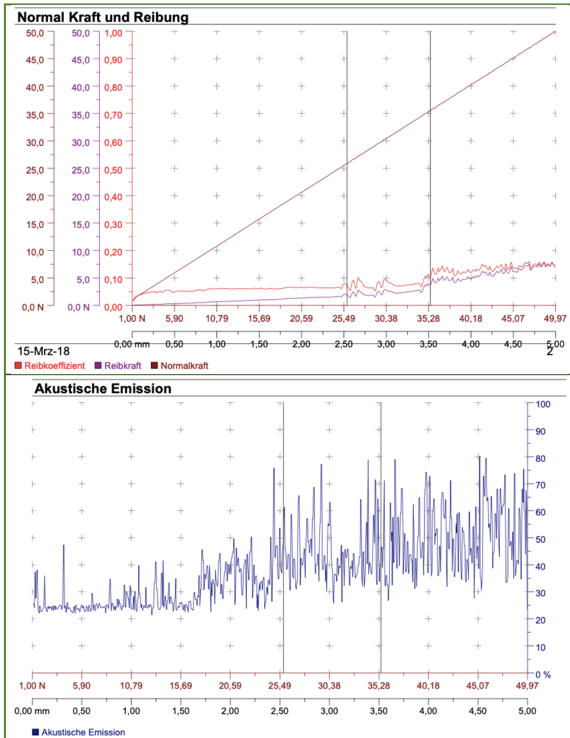
PRILOG P.24: Dijagrami faktora trenja, sile trenja, normalne sile te akustične emisije dobiveni ispitivanjem brazdanjem za uzorak SH-15-T-2, II. mjerenje
