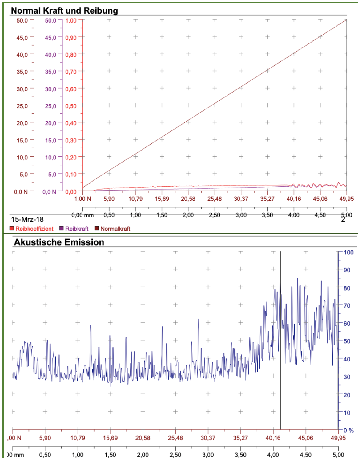
PRILOG P.25: Dijagrami faktora trenja, sile trenja, normalne sile te akustične emisije dobiveni ispitivanjem brazdanjem za uzorak SH-5-C-2, II. mjerenje
