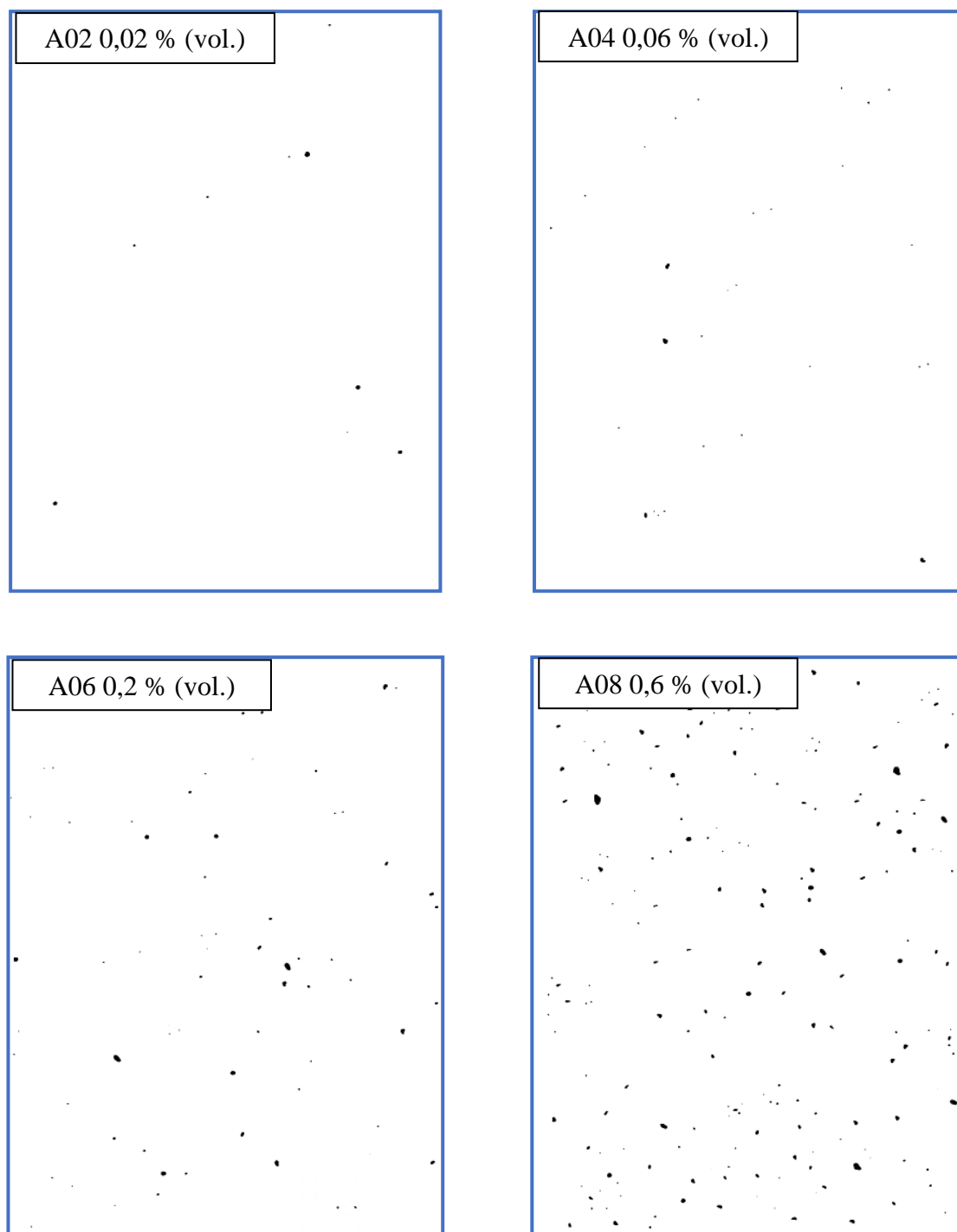
Slika 5.29 Fotomikrografi poroziteta [126]
