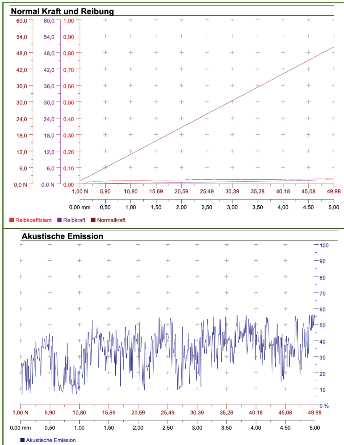
PRILOG P.29: Dijagrami faktora trenja, sile trenja, normalne sile te akustične emisije dobiveni ispitivanjem brazdanjem za uzorak SH-10-B-2, II. mjerenje
