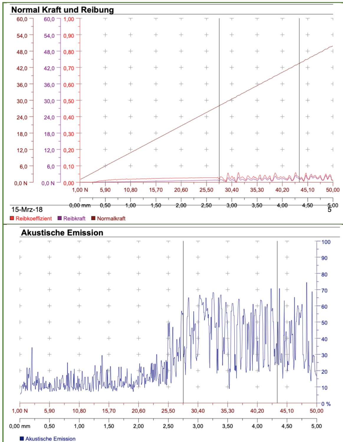
PRILOG P.26: Dijagrami faktora trenja, sile trenja, normalne sile te akustične emisije dobiveni ispitivanjem brazdanjem za uzorak SH-10-C-2, II. mjerenje
