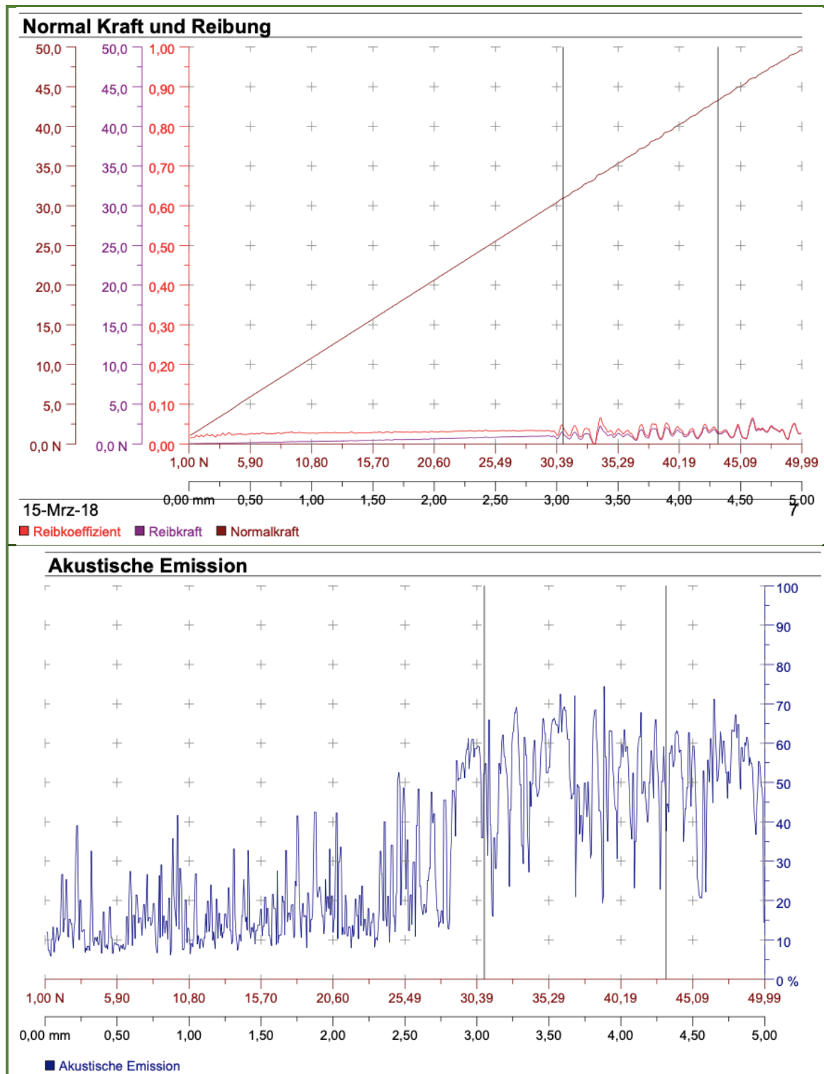
PRILOG P.27: Dijagrami faktora trenja, sile trenja, normalne sile te akustične emisije dobiveni ispitivanjem brazdanjem za uzorak SH-15-C-2, II. mjerenje
