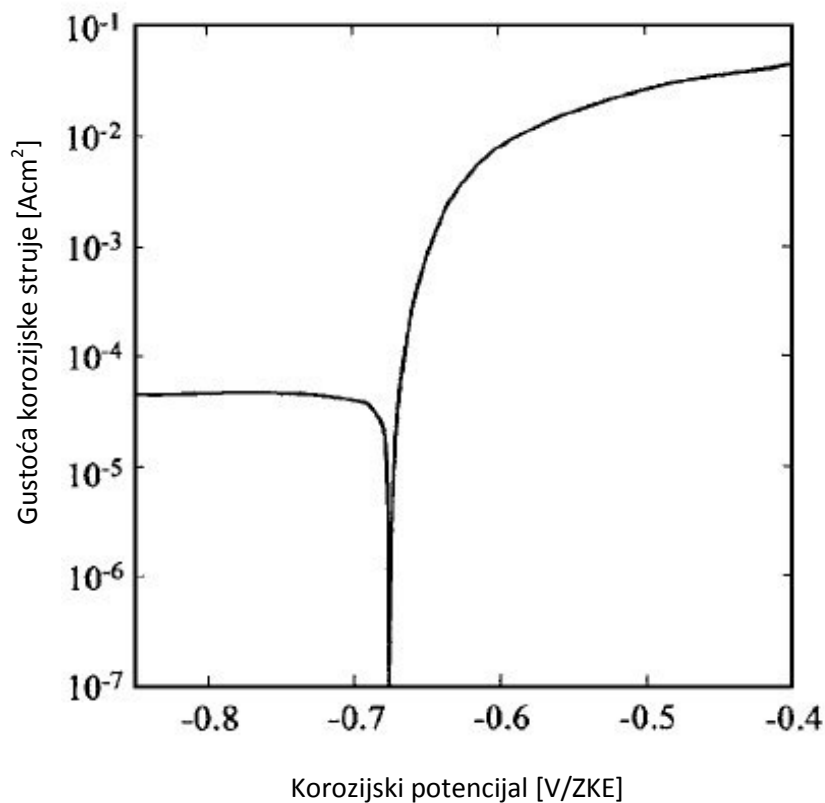
Slika 46: Rezultati elektrokemijskog ispitivanja legure 2024-T351 u otopini koncentracije 1 M NaCl [44]
