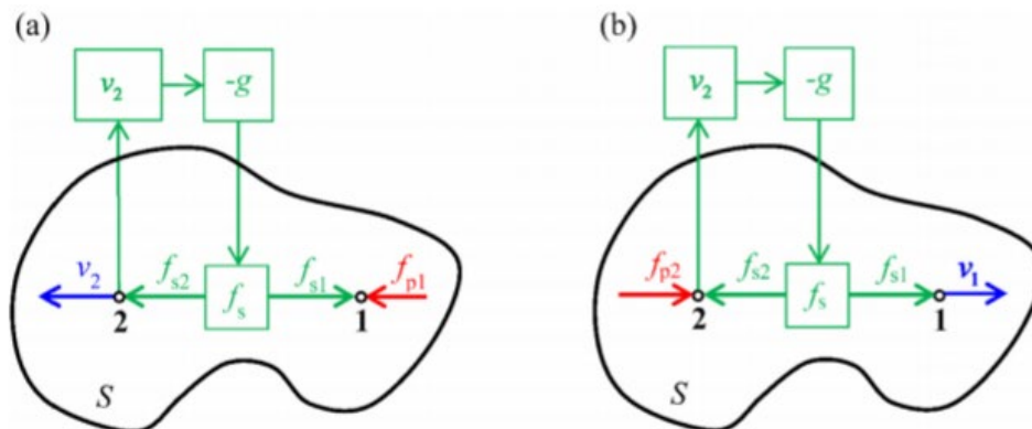
Slika 2: Aktivna linearna konstrukcija (a) uzbuda u točki 1 odziv u točki 2, (b) uzbuda u točki 2 odziv u točki 1
