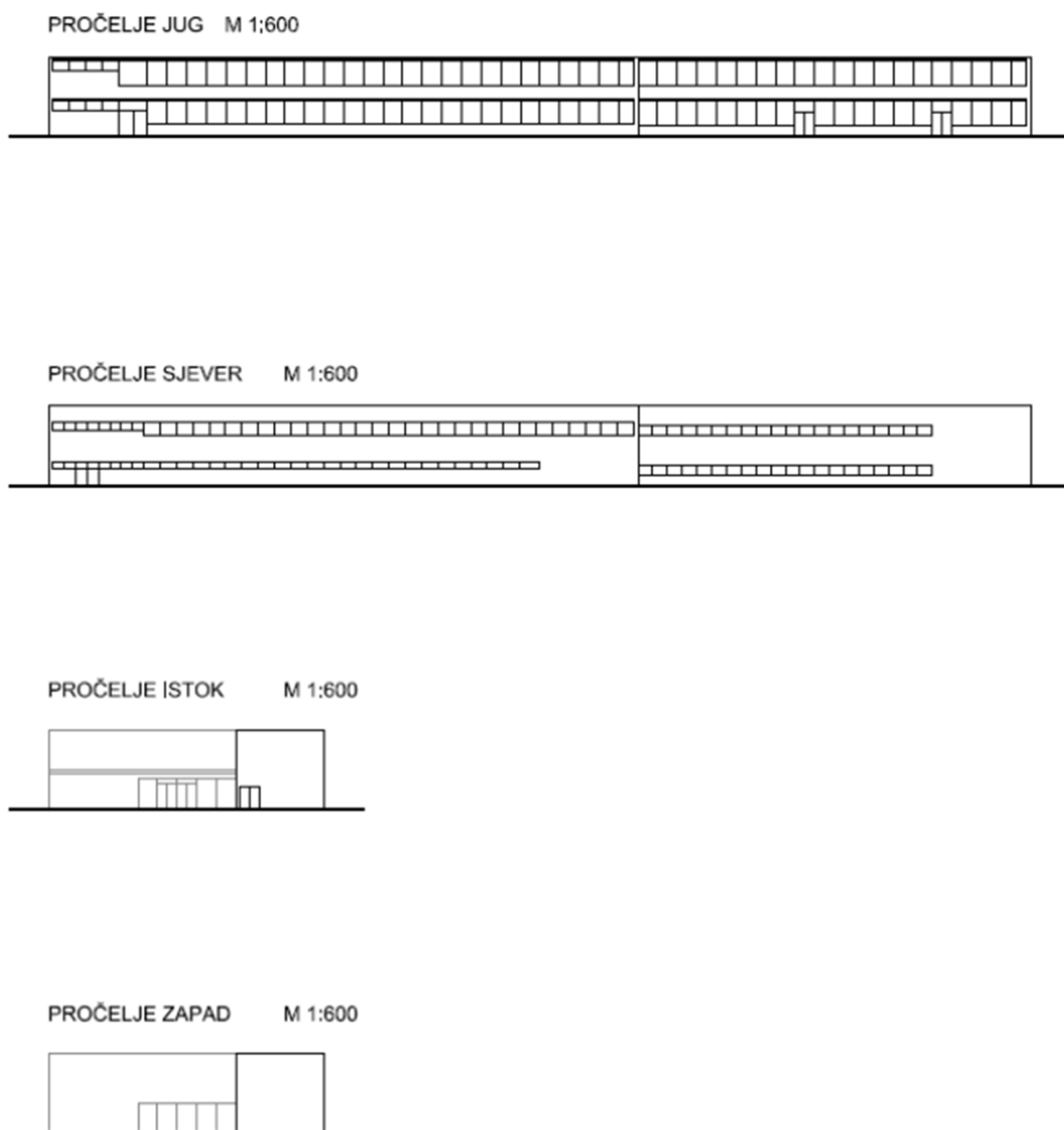
Slika 5. Pročelja nZEB referentne zgrade za obrazovanje
