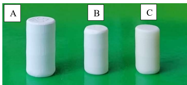
Slika 7.5 Uzorci korišteni u ovom istraživanju: (A) strojno obrađeni \text{Al}_2\text{O}_3 sirovac (uzorak prije sinteriranja), (B) \text{Al}_2\text{O}_3 keramika sinterirana u hibridnoj mikrovalnoj peći i (C) električnoj peći
