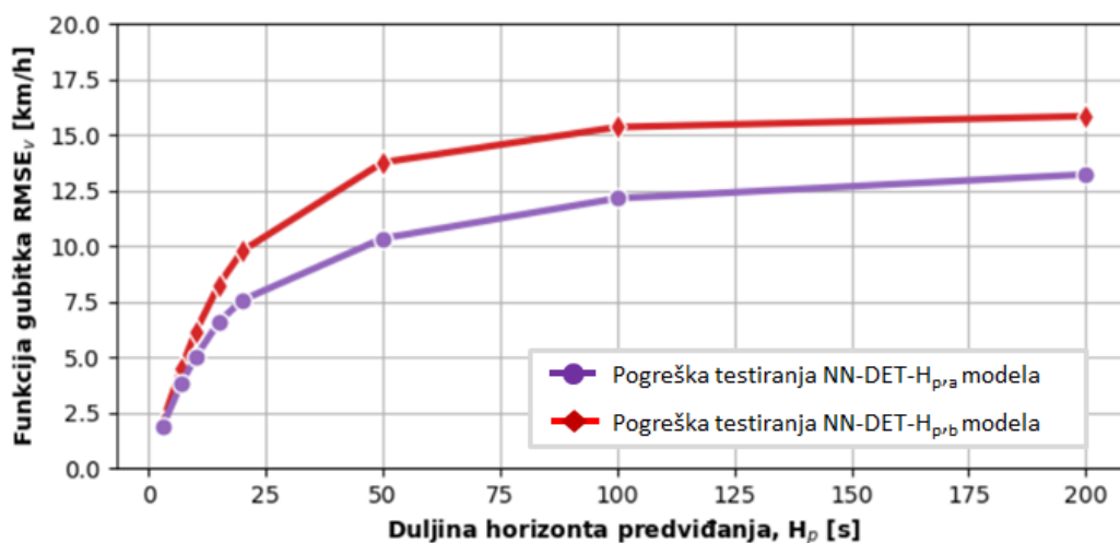
Slika 7-17: Vrijednosti pogreške testiranja RMSE_v za različite duljine horizonta predviđanja H_p i različite prediktivne modele.
