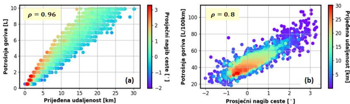
Slika 4-5: Potrošnja goriva u odnosu na a) prijeđenu udaljenost i b) prosječni nagib ceste za kombinirane vozne cikluse (one koji sadrže snimljene mikrocikluse).
