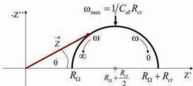
Slika 14. Nyquistov dijagram [10]
