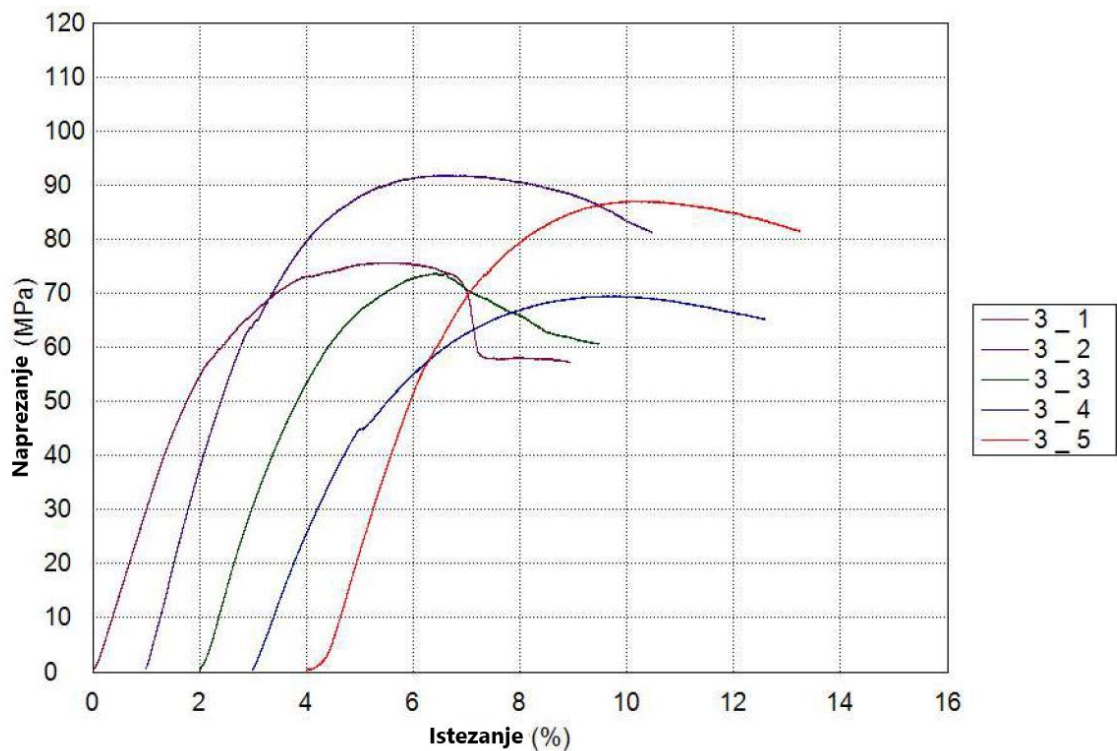
Slika 32. Dijagram savjnoga napreznja – istežanja za LSLLSL konfiguraciju materijala
