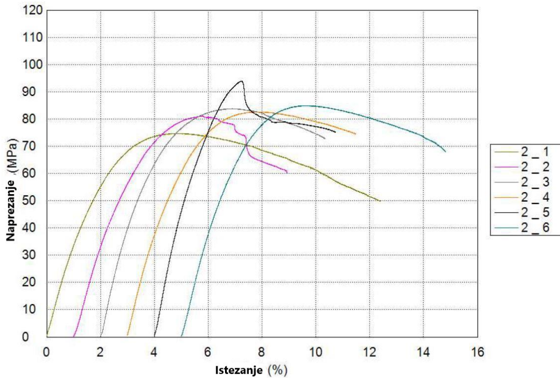
Slika 31. Dijagram savjnoga napreznja – istežanja za LLSSL konfiguraciju materijala
