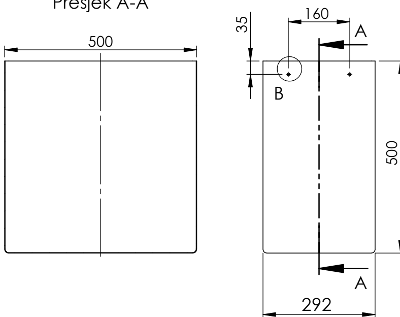
Presjek A-A
