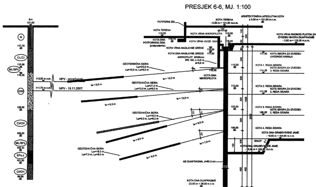
Slika 19. Karakterističan presjek s 4 reda sidara za dio južne strane jame s produbljjenjem
