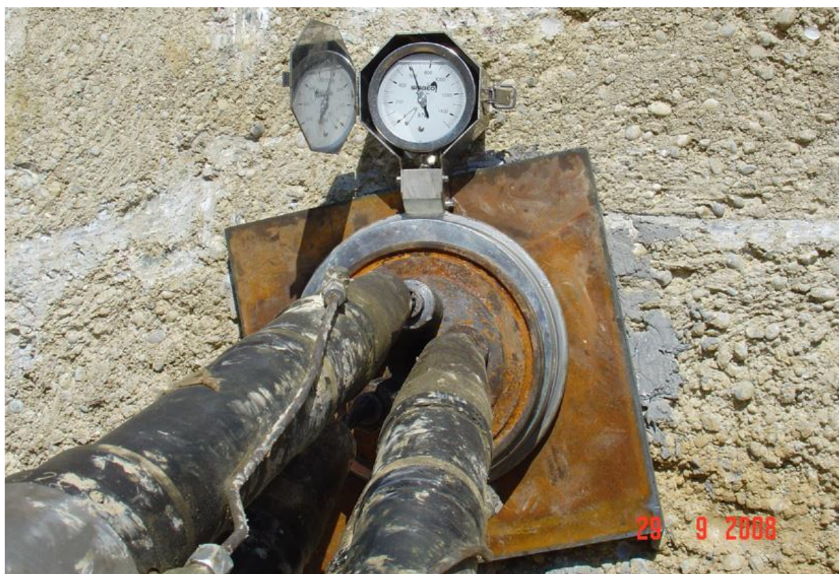
Slika 23. Ugrađeni dinamometar za praćenje sile u sidru [13]
