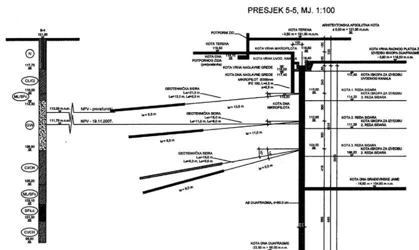
Slika 18. Karakterističan presjek s 3 reda sidara na dijelu južne strane jame bez produbljjenja
