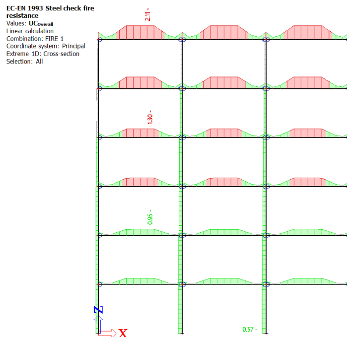
Slika 74 Proračun čeličnih elemenata CS2 na djelovanje požara (Scenarij 4)
