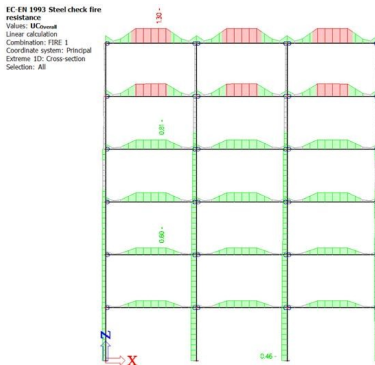
Slika 75 Proračun čeličnih elemenata CS2 na djelovanje požara (Scenarij 1)
