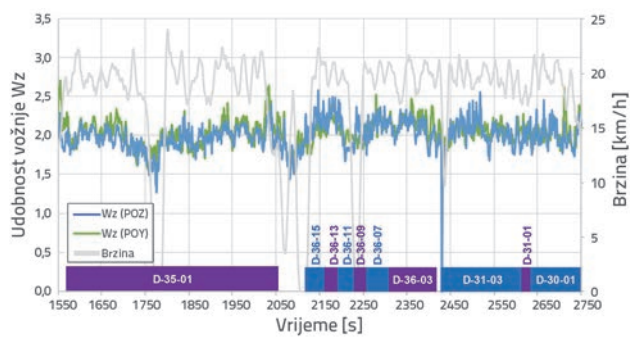
Slika 16. Sperlingov indeks udobnosti vožnje Wz na ispitnoj dionici 2, zapadni kolosijek
