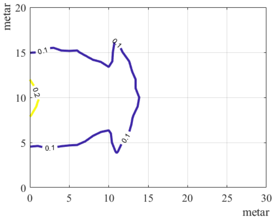
Prilog 12 Polje koeficijenta transmisije za val valne visine 0,6 m i perioda 2,77 s; uronjena grupa propusta (W1) postavljena na koordinati (0,10) i os propusta je paralelna s apcisolom (Slika 63)
