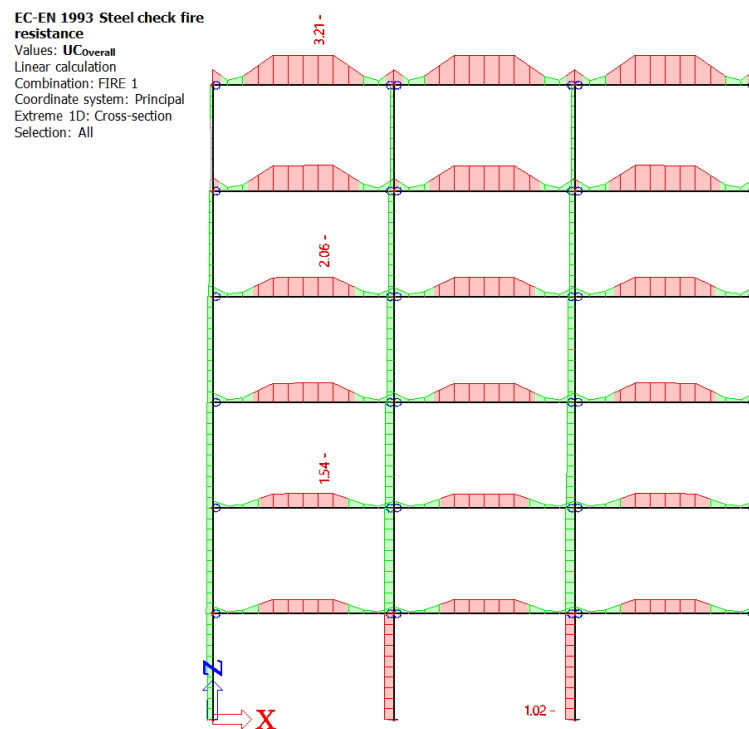
Slika 76 Proračun čeličnih elemenata CS2 na djelovanje požara (Scenarij 6)
