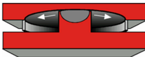
Slika 35.: Primjer konkavnog kliznog ležaja [8]
