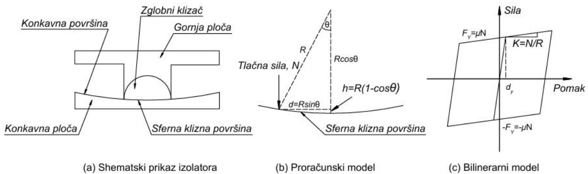
Slika 38.: Model ponašanja izolatora [22]
