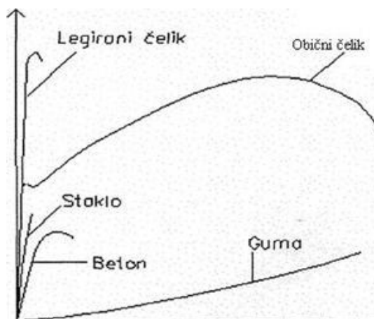
Slika 2., Radni dijagram napreznja materijala[9]
