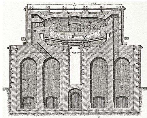
Slika 5., Siemens-Martinova peć, 1895. [12]
