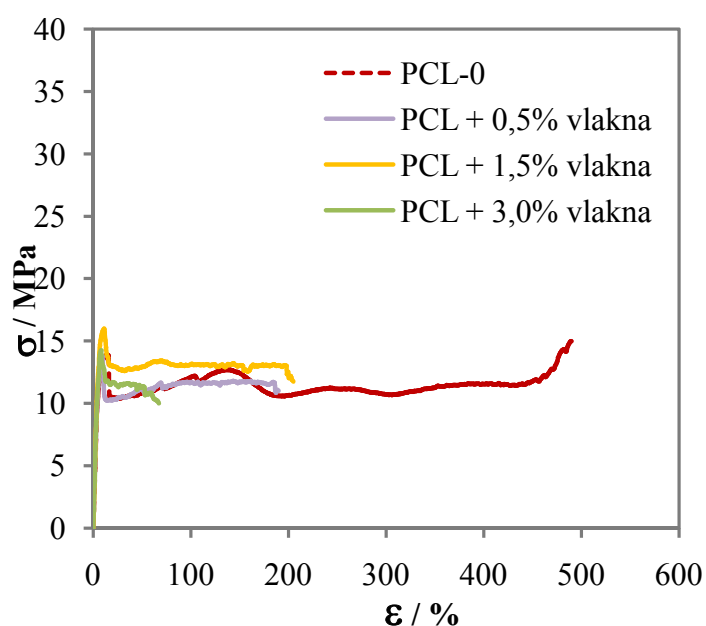
Dijagram 35 – usporedne krivulje napreznja – istezanja za PCL-0 i PCL s dodatkom vlakana
