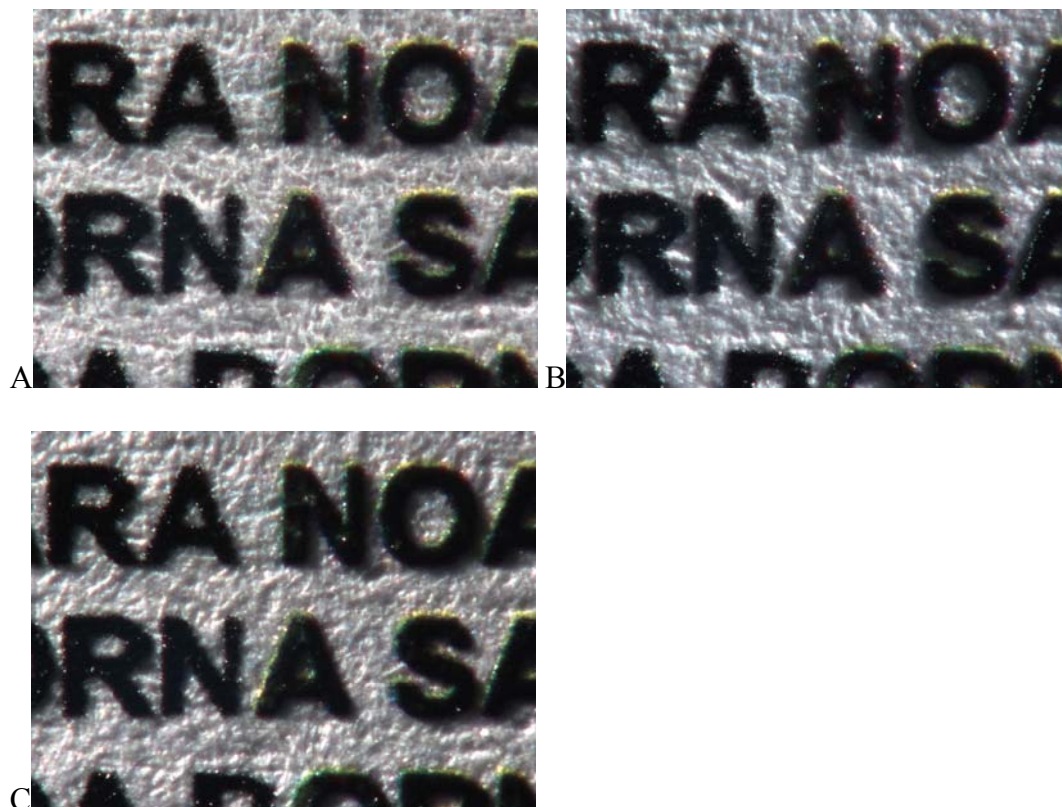
Slika 106 Kontrolirani nanos boje, uvećanje 95 puta. Koso obostrano skaniranje (A), desno koso skaniranje (B) i lijevo koso skaniranje (C).
