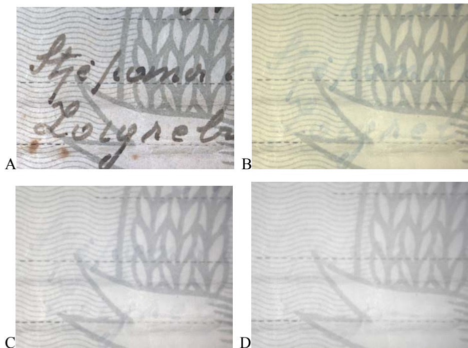
Slika 8 Digitalni zapis svjedočbe iz 1946.godine pod imitacijom bijele svjetlosti (A) i različitim IR valnim duljinama; 715 nm(A), 780 nm(B) i 830 nm(C). Uvećanje 13 puta.
