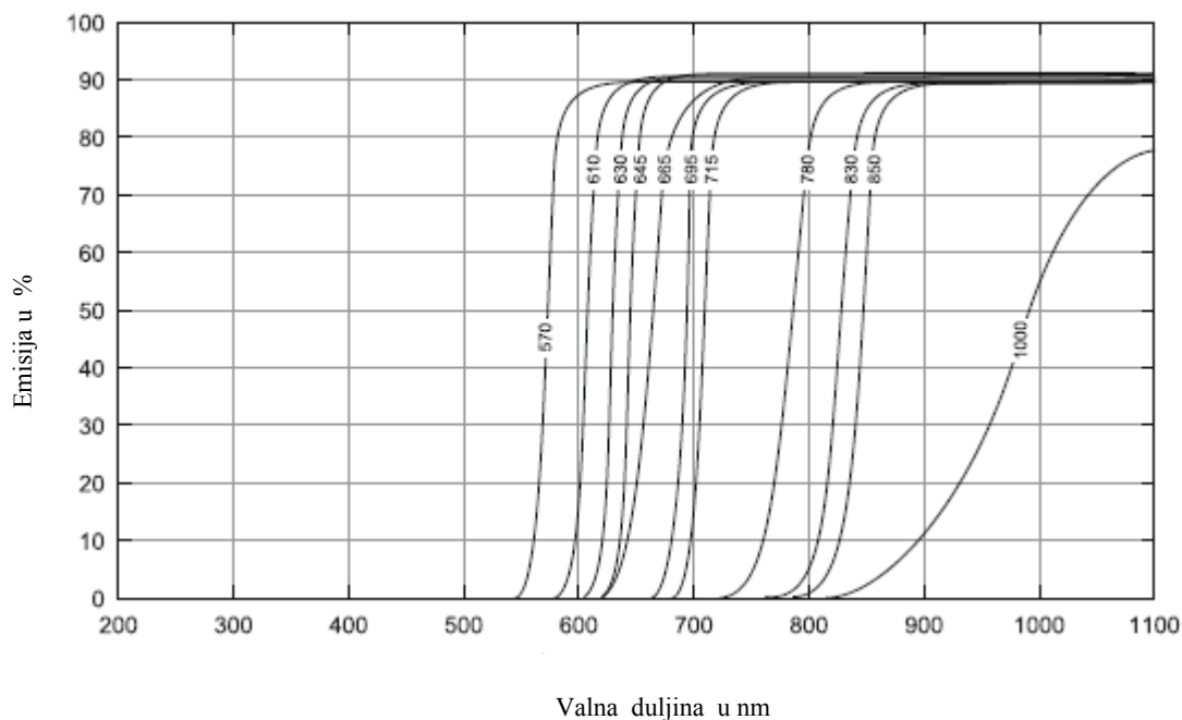
Slika 1 Barijere korištene u eksperimentalnom radu – uređaj docucenter expert
