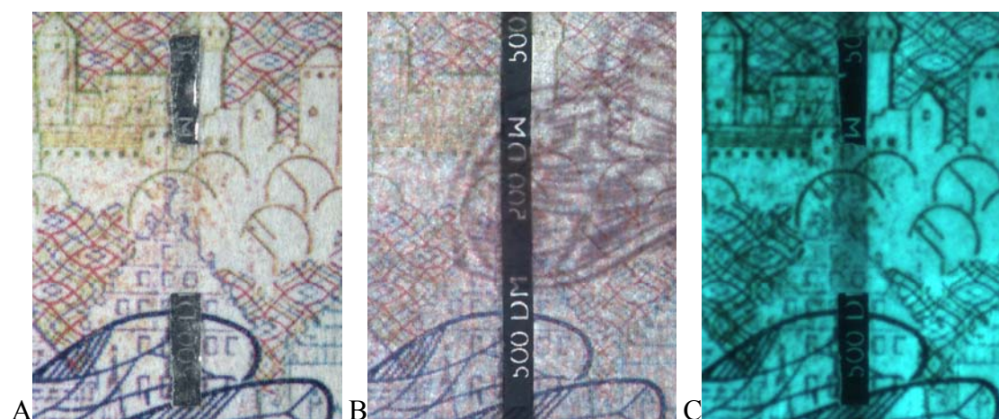
Slika 41. Reprodukcijska zaštitna nit na krivotvorenoj novčanici od 500 DEM, uvećanje 7.4 puta. Imitacija bijelog svjetla (A), propusno svjetlo (B) i ultraljubičasto svjetlo od 365 nm (C).
