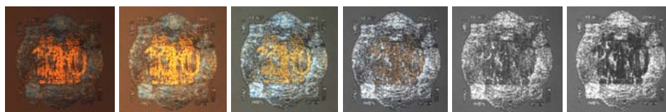
Slika 50. Reprodukcijski hologram na krivotvorenoj novčanici od 100 eura indikatora P13, uvećanje 13 puta. Infracrveno svjetlo od 630,645,715,780,830 i 1000 nm.
