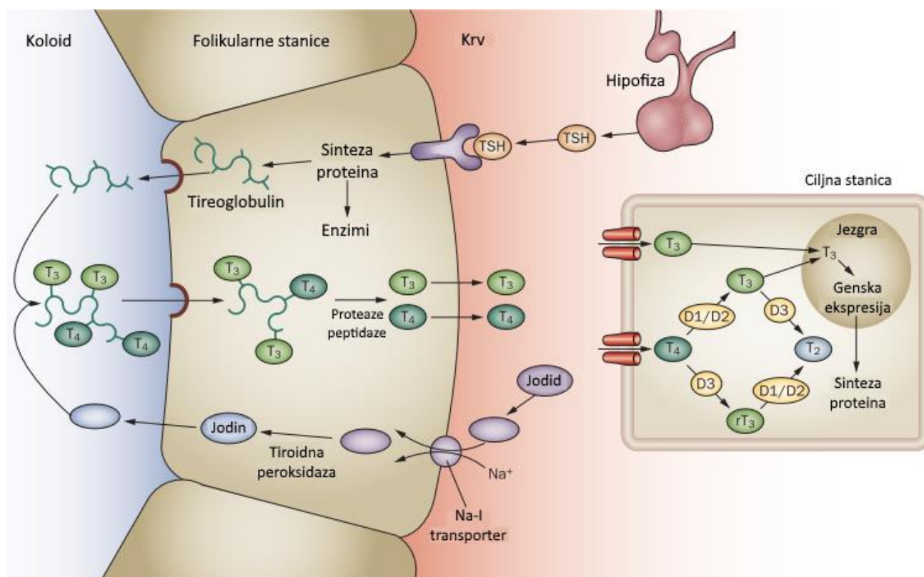
Slika 1. Sinteza tiroidnih hormona. Hormoni štitnjače se sintetiziraju u folikularnim stanicama štitne žlijezde od tirozinskih ostataka unutar molekule tireoglobulina. T4 i T3 zatim se cijepaju i otpuštaju u cirkulaciju. T3, fiziološki aktivni oblik, također nastaje monodejodinacijom iz T4. T4 se konvertira u T3 najčešće tipom 1 dejodinaze. Modificirano prema: Cohen-Lehman J, Dahl P, Danzi S, Klein I. Effects of amiodarone therapy on thyroid function. Nat Rev Endocrinol. 2010;6(1):34–41.
