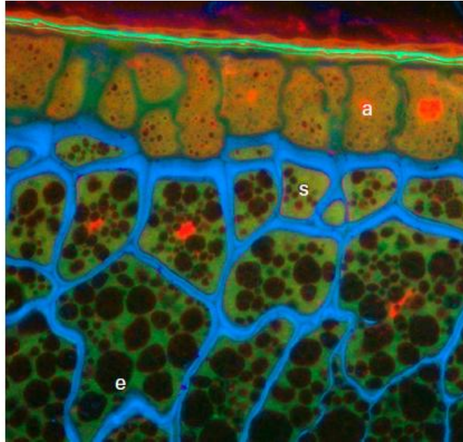
Slika 2. Beta-glukan u staničnoj stijenci obojan plavom bojom. a, aleuron; s, subaleurone; e, endosperm. Preuzeto iz Wang i Ellis (2014), ljubaznošću S.S. Miller, Agriculture and Agri-Food Canada.
