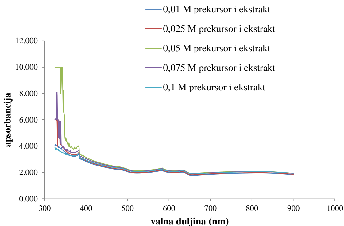
Slika 9. Grafički prikaz UV spektra reakcijskih smjesa
