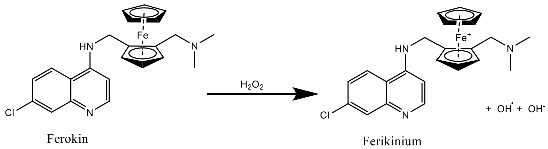
Slika 11. Interkonverzija između ferokina i ferikininiuma s nastankom hidroksilnih radikala.
