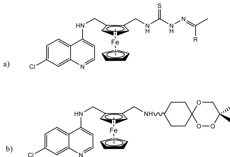
Slika 13. a) ferokin tiosemikarbazon; b) trioksaferokin.
