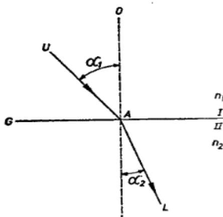
Slika 6. Lom svjetlosti na granici dva sredstva (preuzeto iz Winterhalter i sur., 1990)
