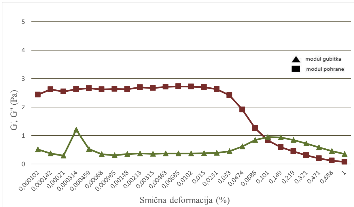
Slika 14. Ovisnost modula pohrane ( G' ) i modula gubitka ( G'' ) nanoemulzije s 0,2% gelan gume (NG3) o smičnoj deformaciji nakon miješanja s ATS-om pri temperaturi od 34°C. Mjerenja su provedena u duplikatu.
