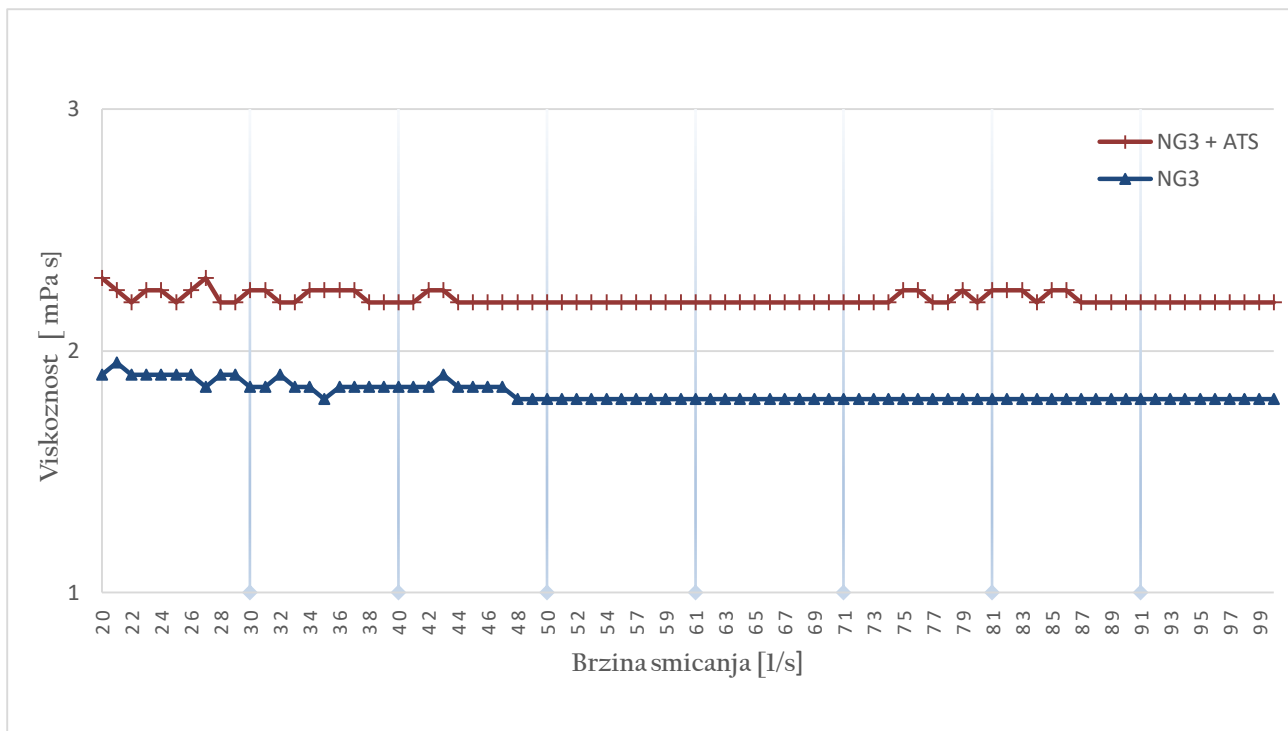
Slika 9. Krivulje viskoznosti nanoemulzije s 0,2% gelan gume prije (NG3) i nakon miješanja s ATS-om (NG3+ATS). Sva mjerenja su provedena u duplikatu.
