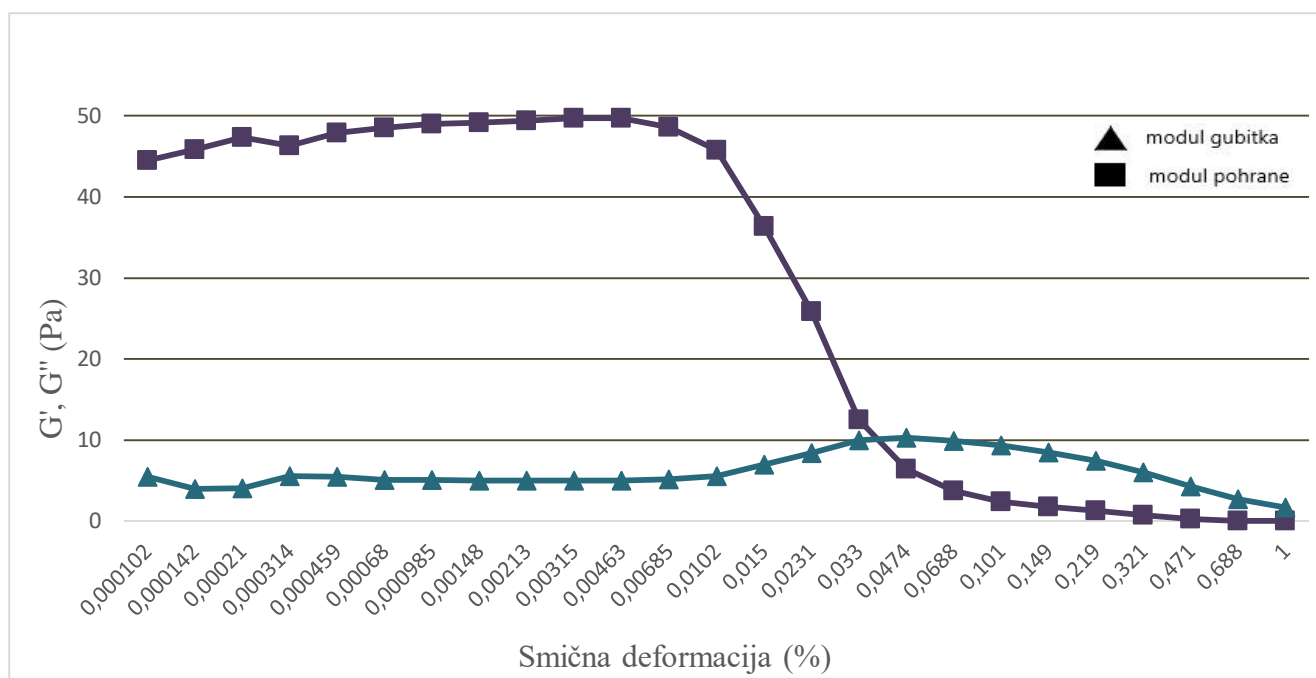
Slika 15. Ovisnost modula pohrane ( G' ) i modula gubitka ( G'' ) nanoemulzije s najvećim udjelom gelan gume (0,4%; NG4) o smičnoj deformaciji nakon miješanja s ATS-om pri temperaturi od 34°C. Mjerenja su provedena u duplikatu.
