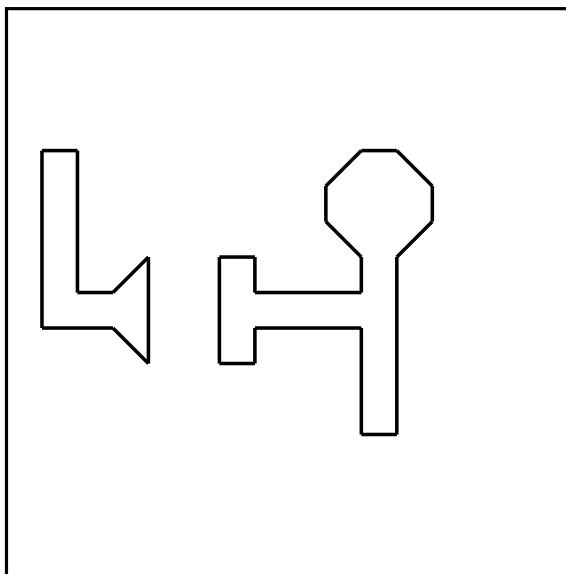
Slika 2.8: Zadane komponente
