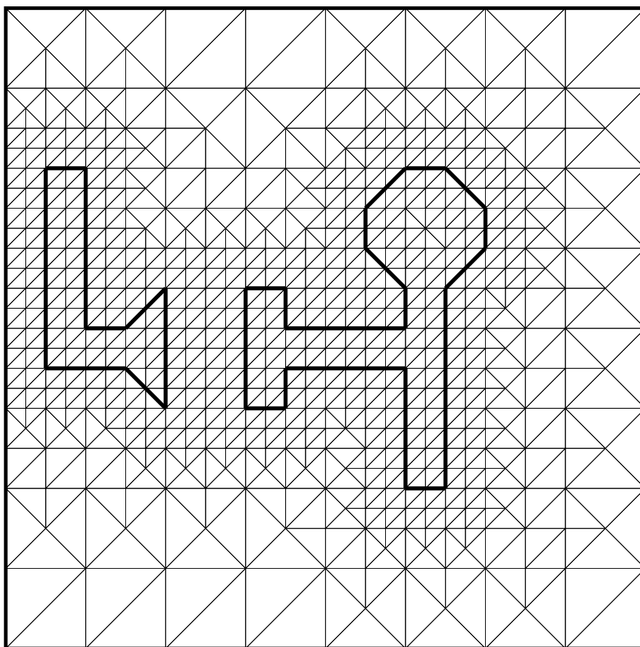
Slika 2.22: Generirana triangulacija
