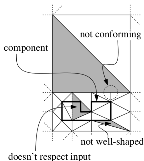
Slika 2.2: Svojstva triangulacije
