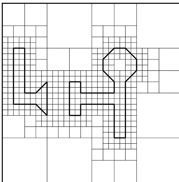
Slika 2.13: Završna podjela
