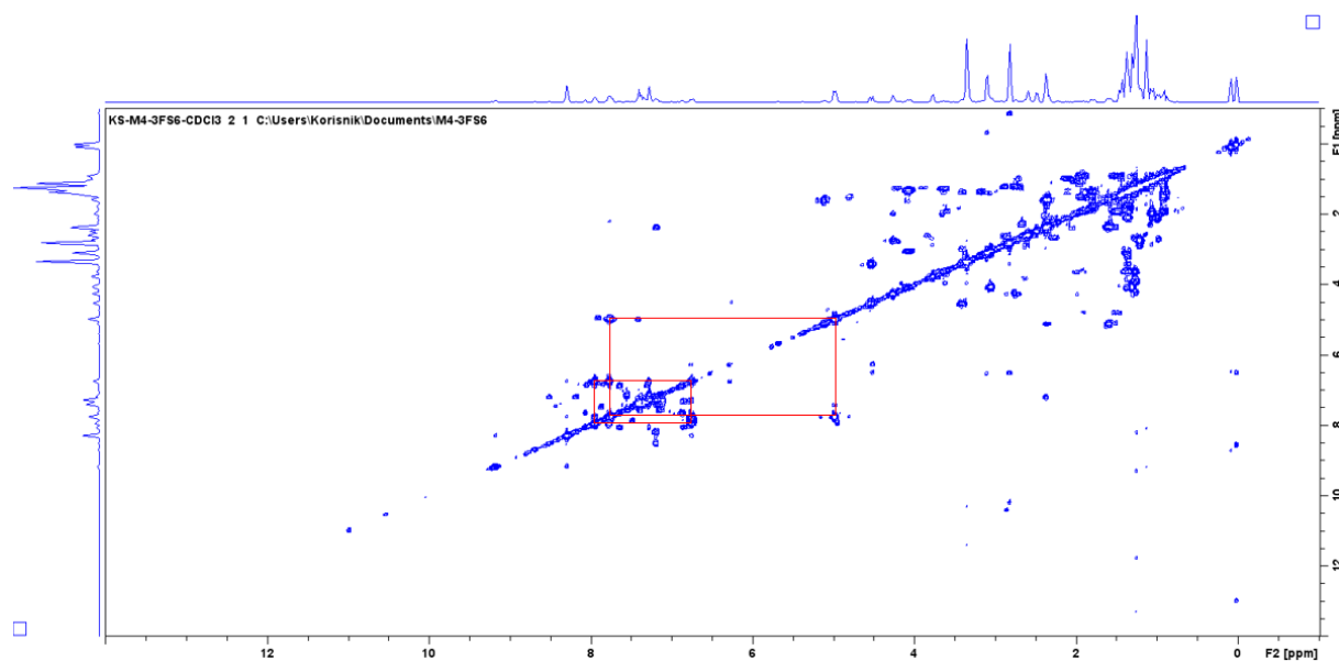
Slika 47. Spektar COSY makrozona, snimljen u CDCl 3 pri 298 K.
