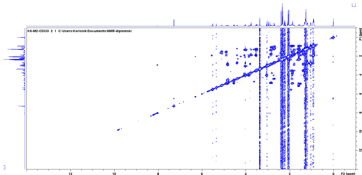
Slika 26. Spektar COSY međuprodukta M2 , snimljen u \text{CDCl}_3 pri 298 K.
