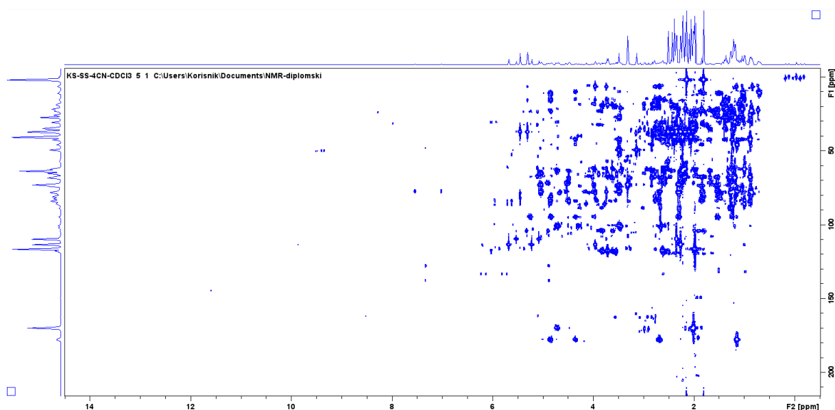
Slika 32. Spektar HMBC adukta M4''CN snimljen u \text{CDCl}_3 pri 298K.
