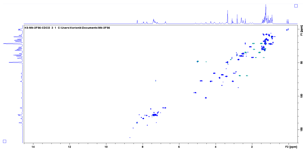
Slika 48. Spektar HSQC makrozona, snimljen u CDCl 3 pri 298 K.
