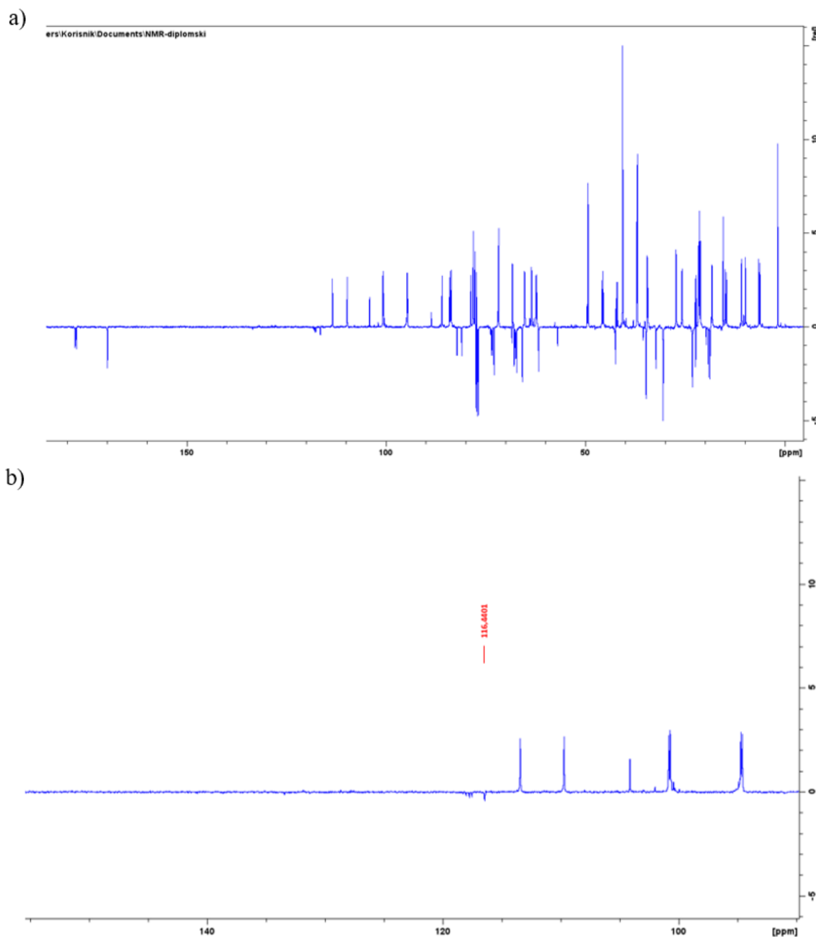
Slika 30. a) spektar DEPT-Q , b) uvećani dio DEPT-Q adukta M4''CN , snimljen u \text{CDCl}_3 pri 298K.
