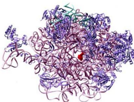
Slika 6. Položaj eritromicina u izlaznom tunelu, 23S rRNA prikazana je svijetloljubičastom bojom, 5S rRNA zelenom bojom, ribosomski proteini tamnoljubičastom bojom, a eritromicin crvenom bojom. 15
