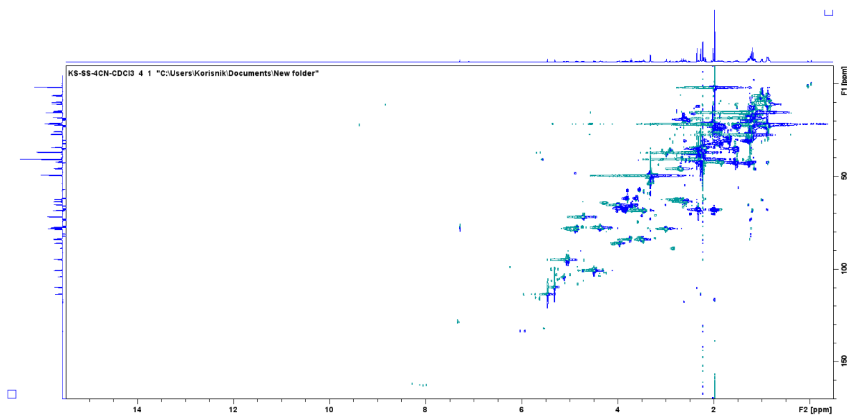
Slika 31. Spektar HSQC adukta M4''CN snimljen u \text{CDCl}_3 pri 298K.
