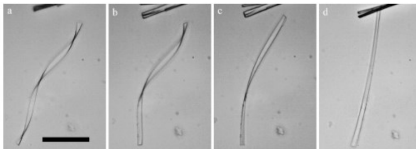
Slika 8. Vraćanje uvijenog kristala 9-antracencarboxilne kiseline nakon uklanjanja svjetlosnog podražaja; (a) odmah po uklanjanju svjetlosnog podražaja, (b) 3 min kasnije, (c) 4,5 min kasnije, (d) 11,5 min kasnije. Slika preuzeta i prilagođena prema izvoru. 21
