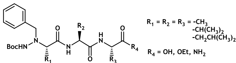
Slika 1. Priprava peptidomimetika s N α -Bn-L-hidrazino-derivatima
