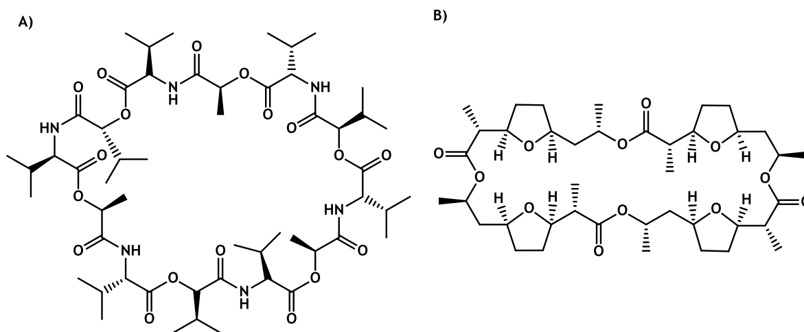
Slika 9. Depsipectidni ionofori; A) Valinomycin, B) Nonaktin
