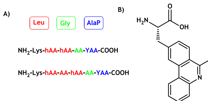
Slika 3. A) Serija peptidomimetika s uzastopnom i naizmjeničnom raspodjelom nezaštićene hidrazino-kiseline (hAaa), B) neprirodna aminokiselina, fenantridinil-L-alanin (AlaP)
