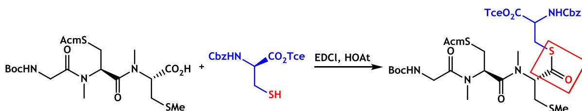
Slika 12. Metoda priprave tiodepsipeptida
