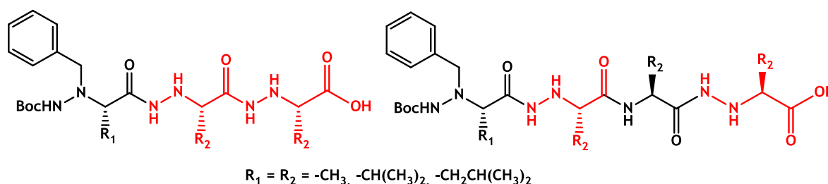
Slika 2. Priprava peptidomimetika s uzastopnom i naizmjeničnom raspodjelom nezaštićene α-hidrazino-kiseline
