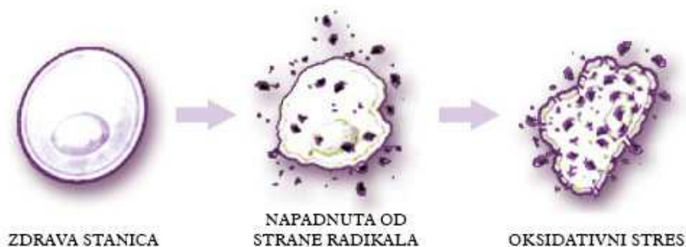
Slika 1. Oksidativni stres prouzrokovan slobodnim radikalima
