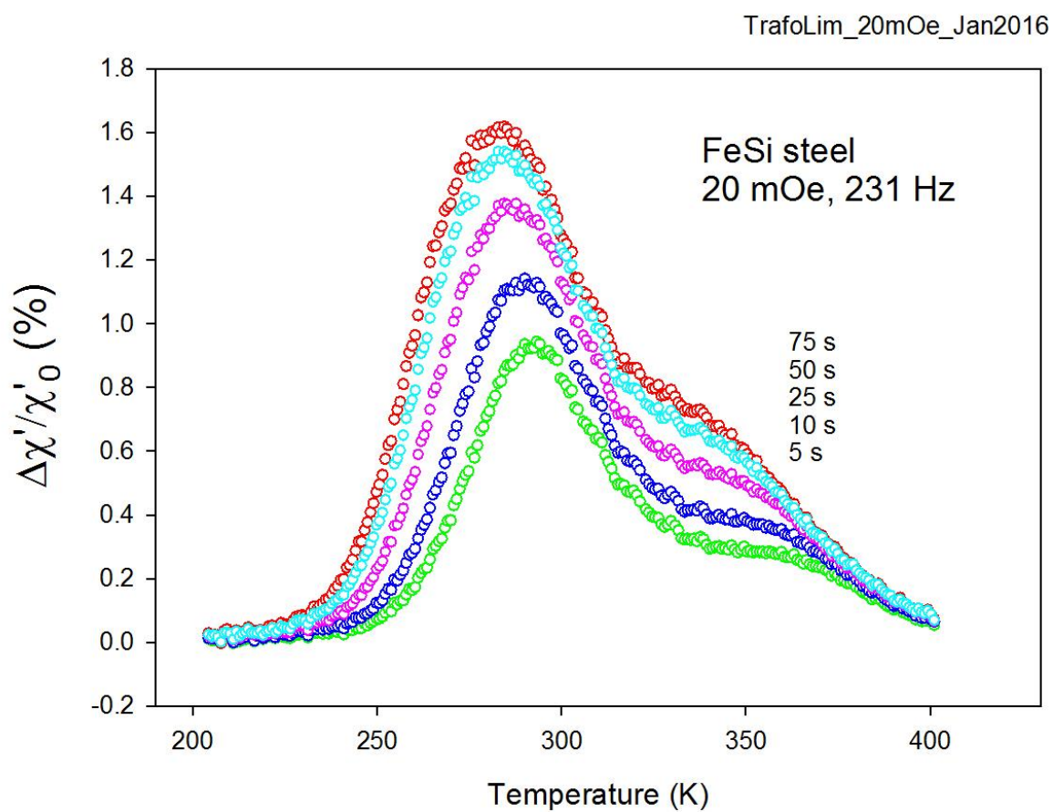
Slika 25. MAE mjerenja za trafoLim
