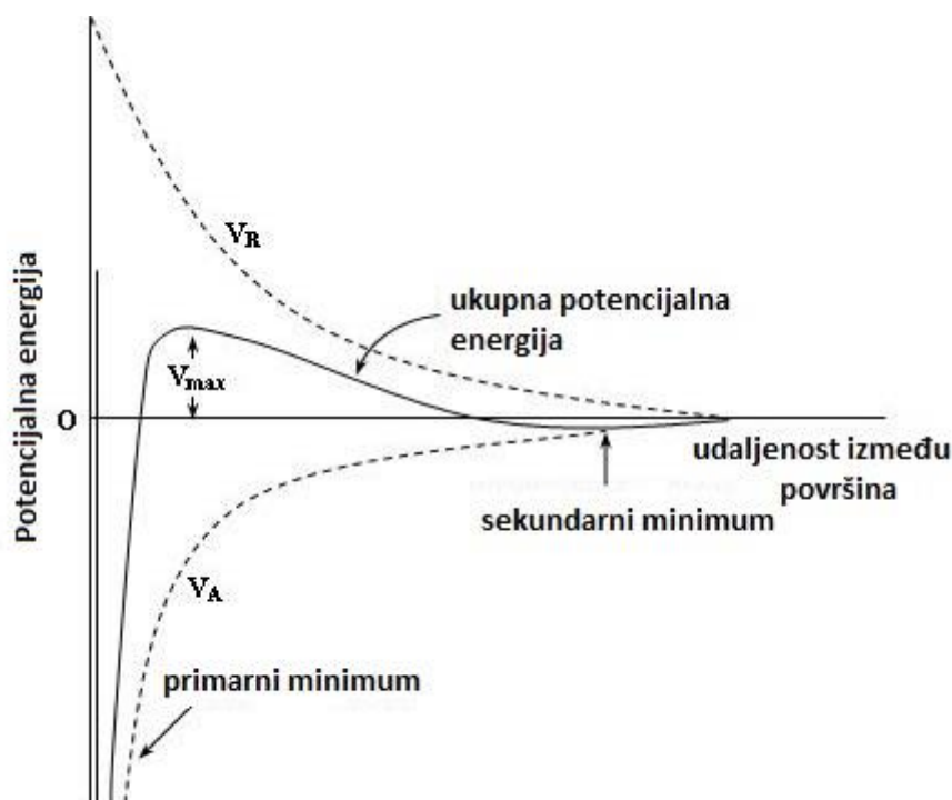
Slika 2. Shematski prikaz potencijala Van der Waalsovih privlačnih sila, potencijala elektrostatskih odbojnih sila, i njihova kombinacija kao funkcija udaljenosti od površine sferične čestice
