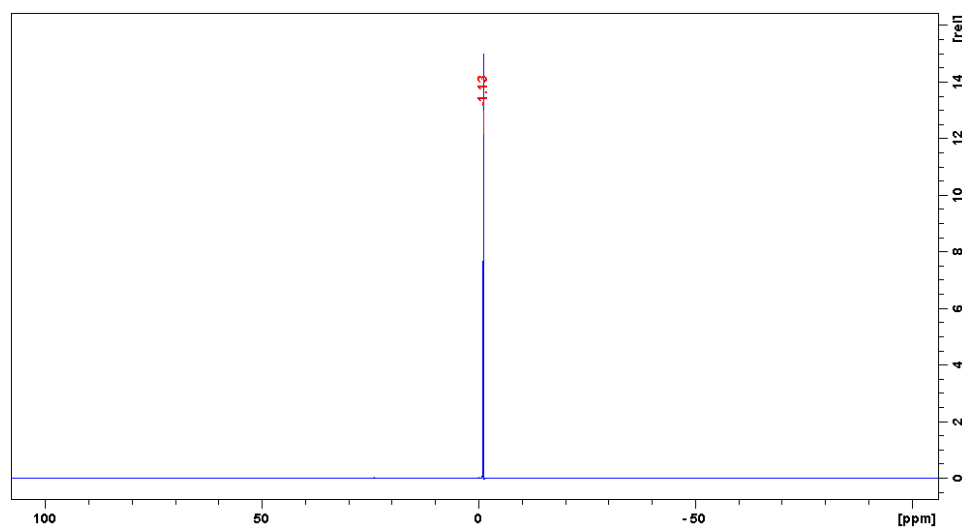
Slika D2. 31 P NMR spektar liganda DL1 u DMSO- d 6
