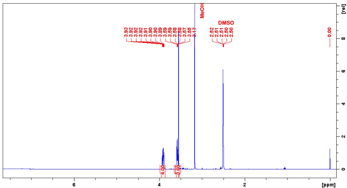
Slika D1. 1 H NMR spektar liganda DL1 u DMSO- d 6
